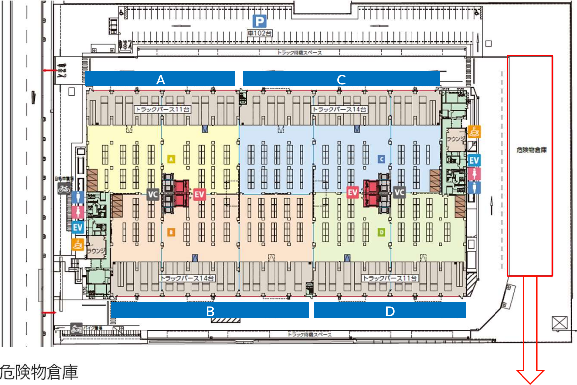
1階 | 配置図・平面図
