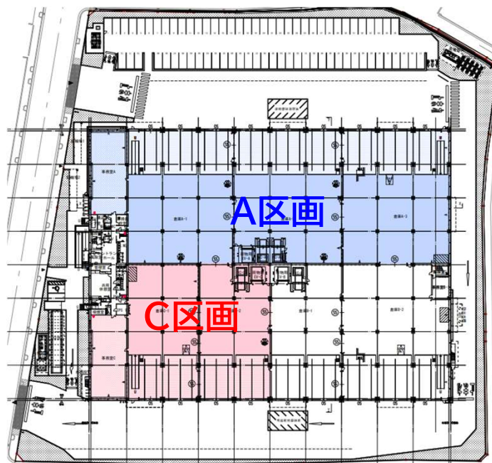
1階 | 配置図・平面図
